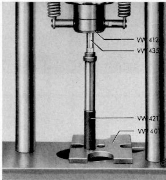
3 - Buchse für Kupplungsfußhebelwelle auf VW-Reparaturpresse in Verbindung mit VW 412, VW 435, VW 421 und VW 401 einpressen.
