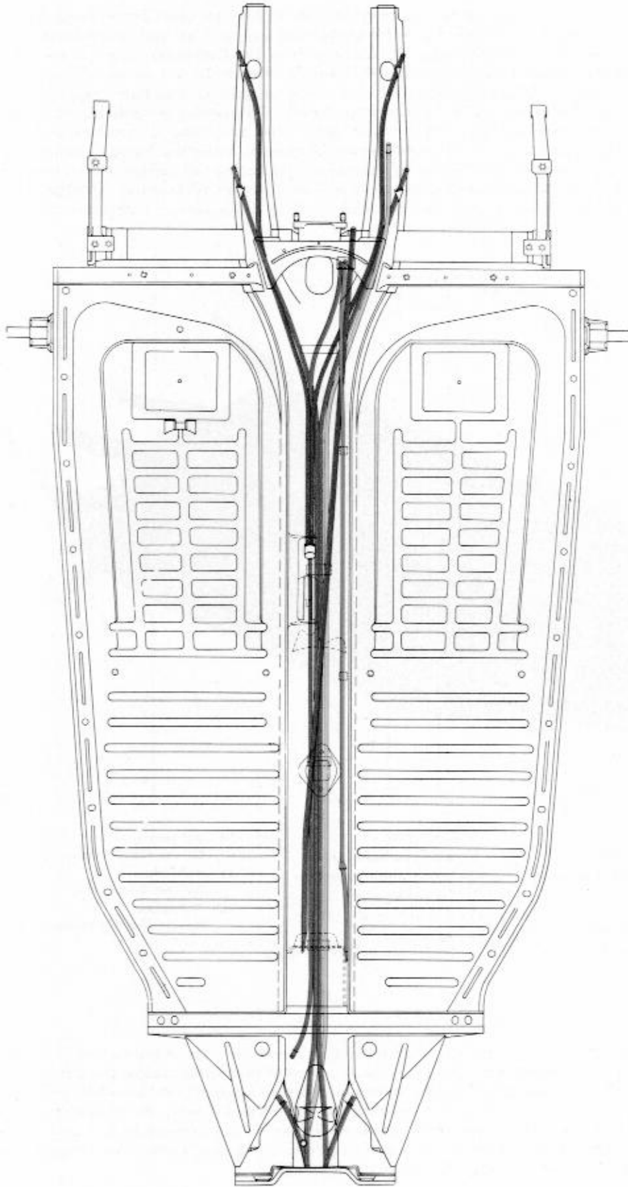
Rahmen mit Führungsrohren und Kraftstoffleitung (Standardmodell)
